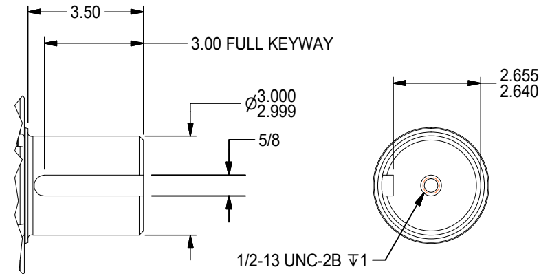
D2 Output Shaft \phi 3.00 X 5/8" Keyway
